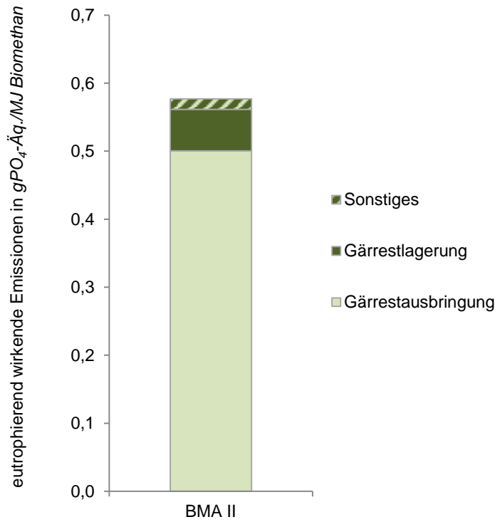
Abbildung 7-21: Spezifische eutrophierend wirkende Emissionen der BMA II in gPO 4 -Äq./MJ Biomethan
