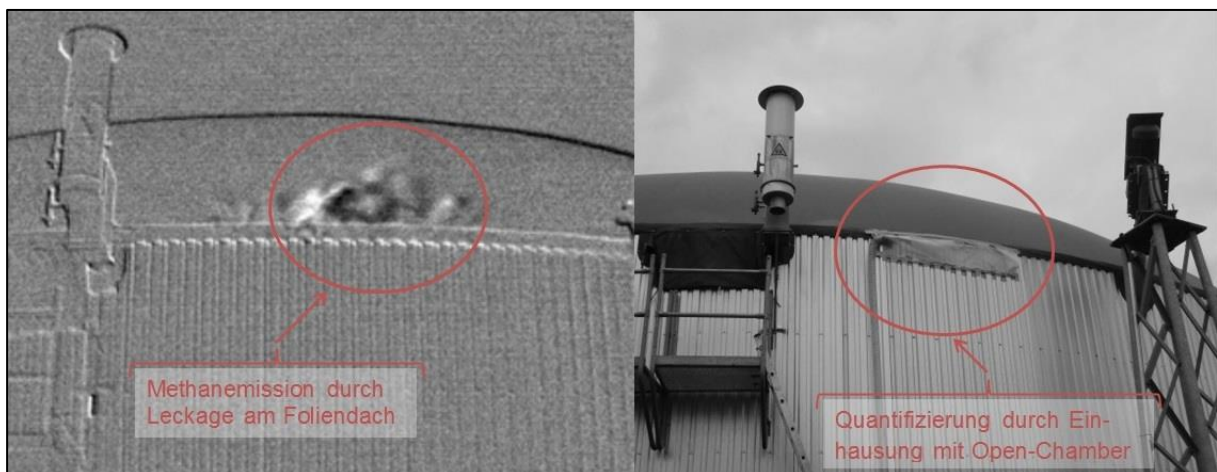
Abbildung 5-13: Leckage am Übergang der Dachfolie zur Behälterwand eines Fermenters
