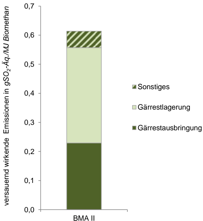
Abbildung 7-18: Spezifische versauernd wirkende Emissionen der BMA II in gSO 2 -Äq./MJ Biomethan
