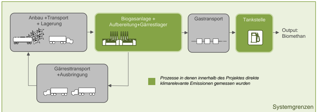
Abbildung 7-2: Systemgrenzen der Bilanzierung am Beispiel der BMA I
