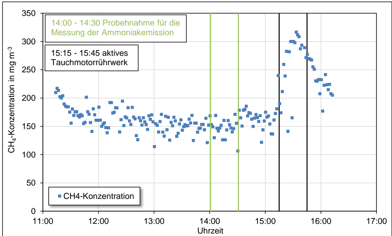
Abbildung 5-20: Einfluss von Rührintervallen auf die Methanemission
