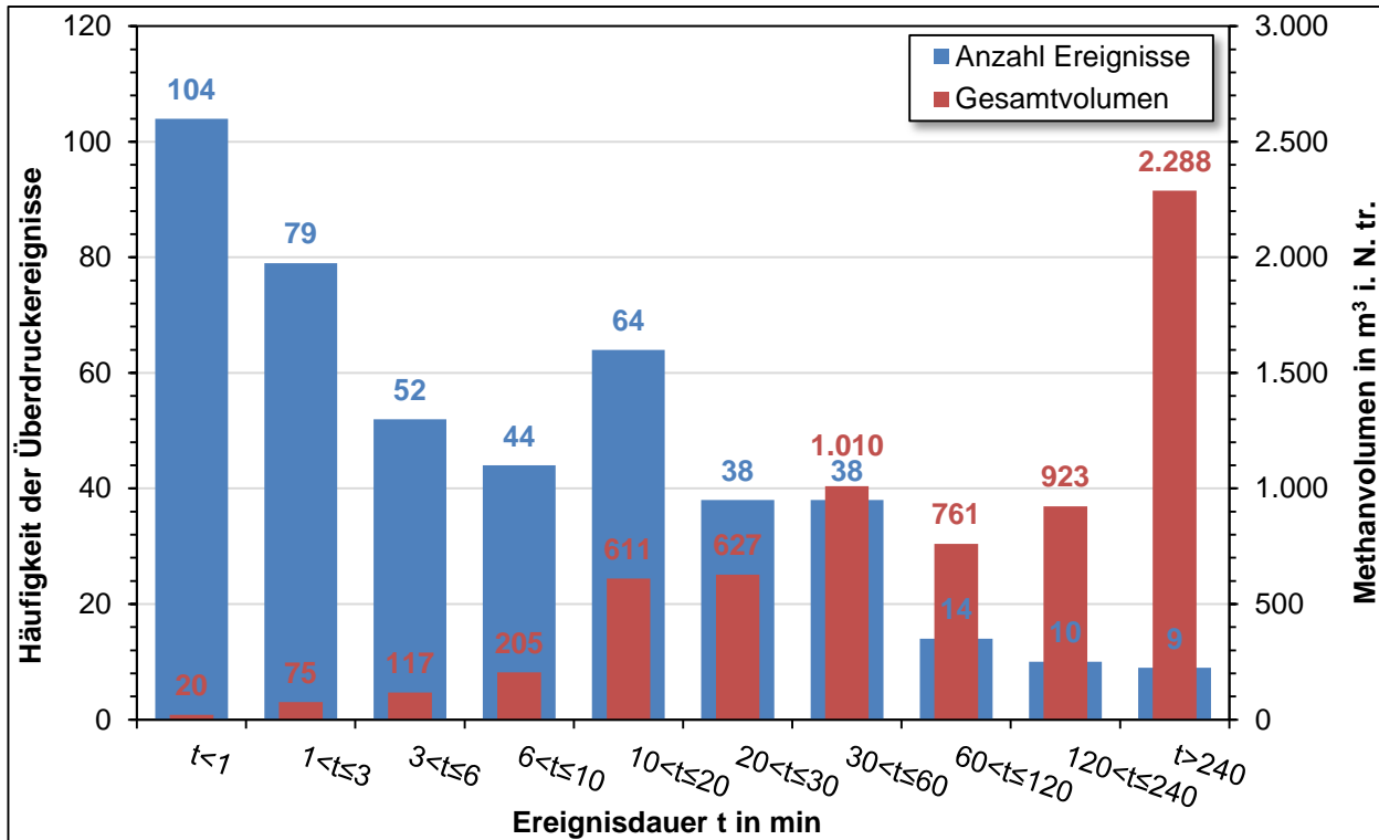
Abbildung 5-32: Dauer und emittiertes Methanvolumen von Überdruckereignissen; Einteilung in Ereignisklassen nach der Dauer der Ereignisse
