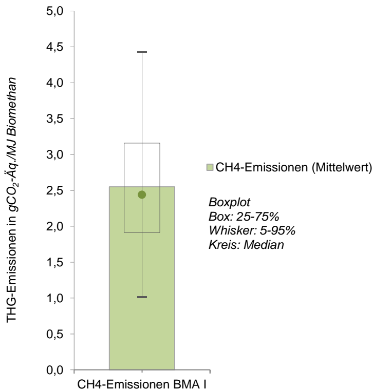
Abbildung 7-7: Treibhausgaspotential der gemessenen CH 4 -Emissionen der BMA I in gCO 2 -Äq./MJ Biomethan
