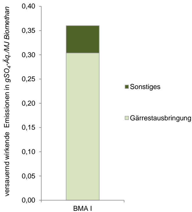
Abbildung 7-17: Spezifische versauernd wirkende Emissionen der BMA I in gSO 2 -Äq./MJ Biomethan
