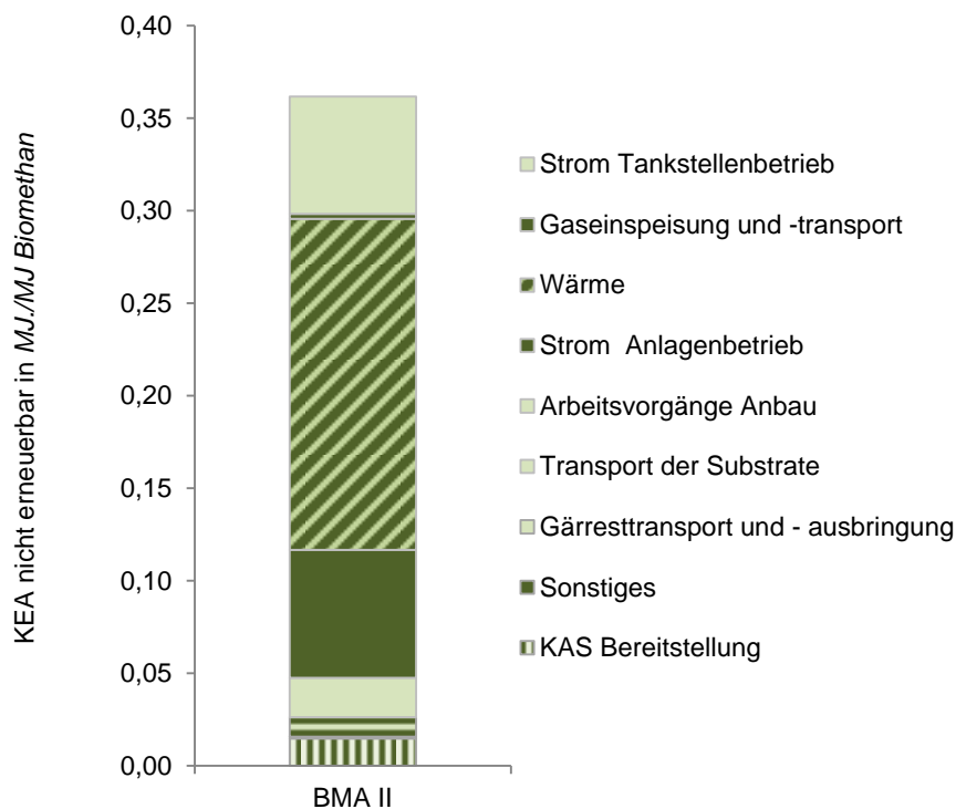
Abbildung 7-24: Kumulierter nicht erneuerbarer Energieaufwand der BMA II in MJ/MJ Biomethan
