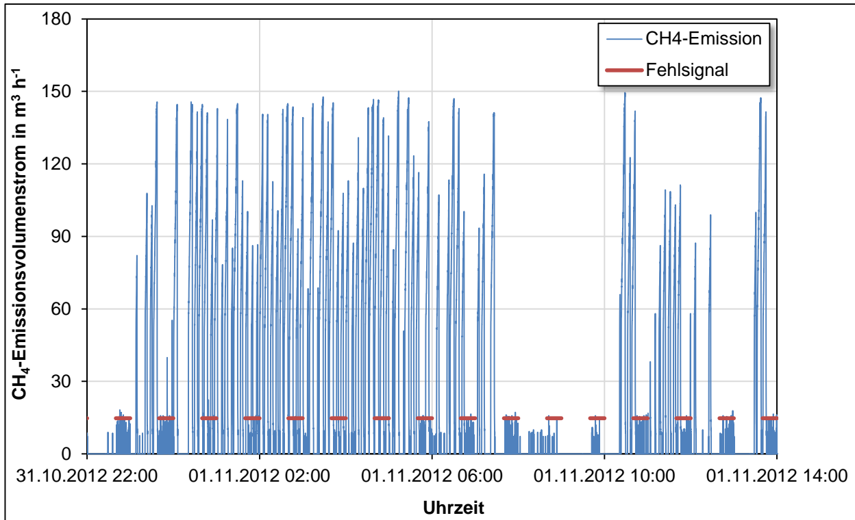
Abbildung 5-29: Auslösen der ÜUDS am Nachgärer 1 (2. Stufe) der Anlage A am 31.10. und 01.11.2012 mit unbekannter Ursache
