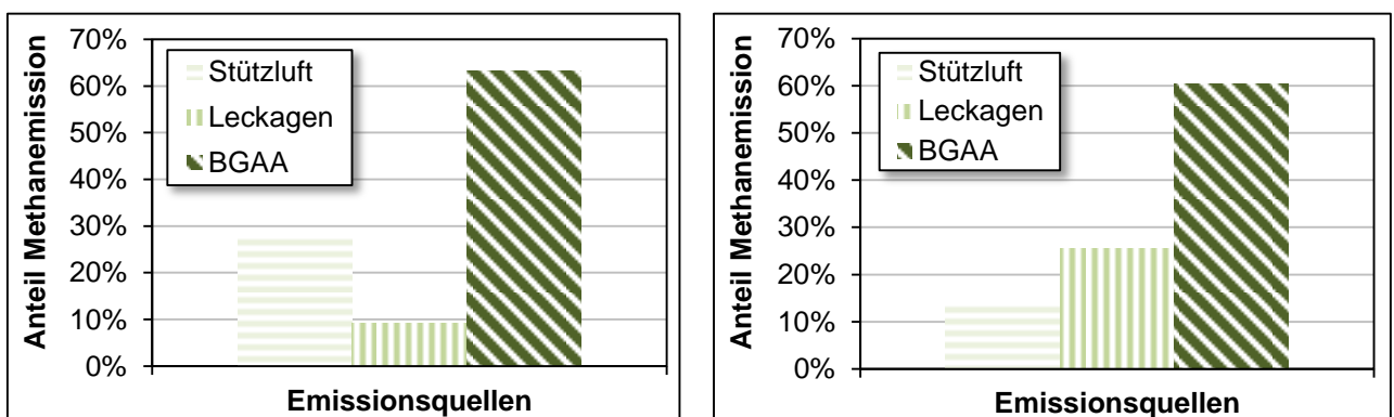
Abbildung 5-10: Beitrag der Quelltypen Leckagen, Stützluft und BGAA zur Gesamtmethanemission in Messphase II (links) und Messphase III (rechts)
