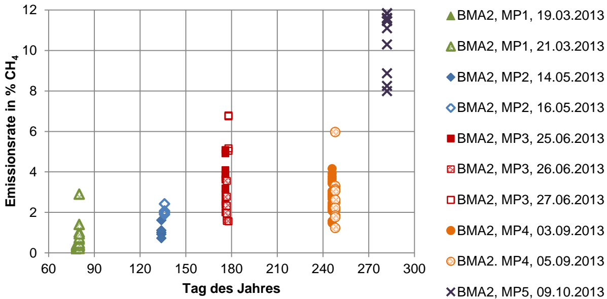
Abbildung 5-45: Viertelstundenwerte der Messkampagnen dargestellt im Jahresverlauf
