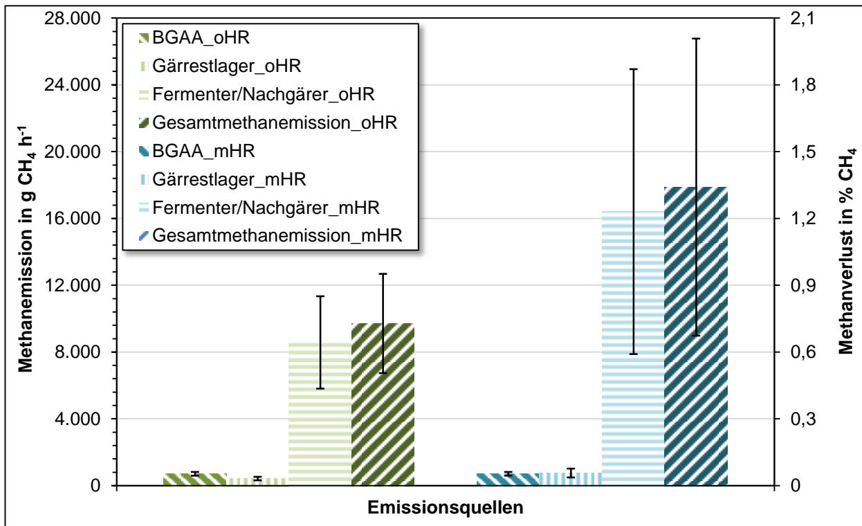
Abbildung 5-18: Mit Vor-Ort-Methode gemessene Emissionen (links) und mit Emissionsfaktoren hochgerechnete Emissionen (rechts) der MP IV
