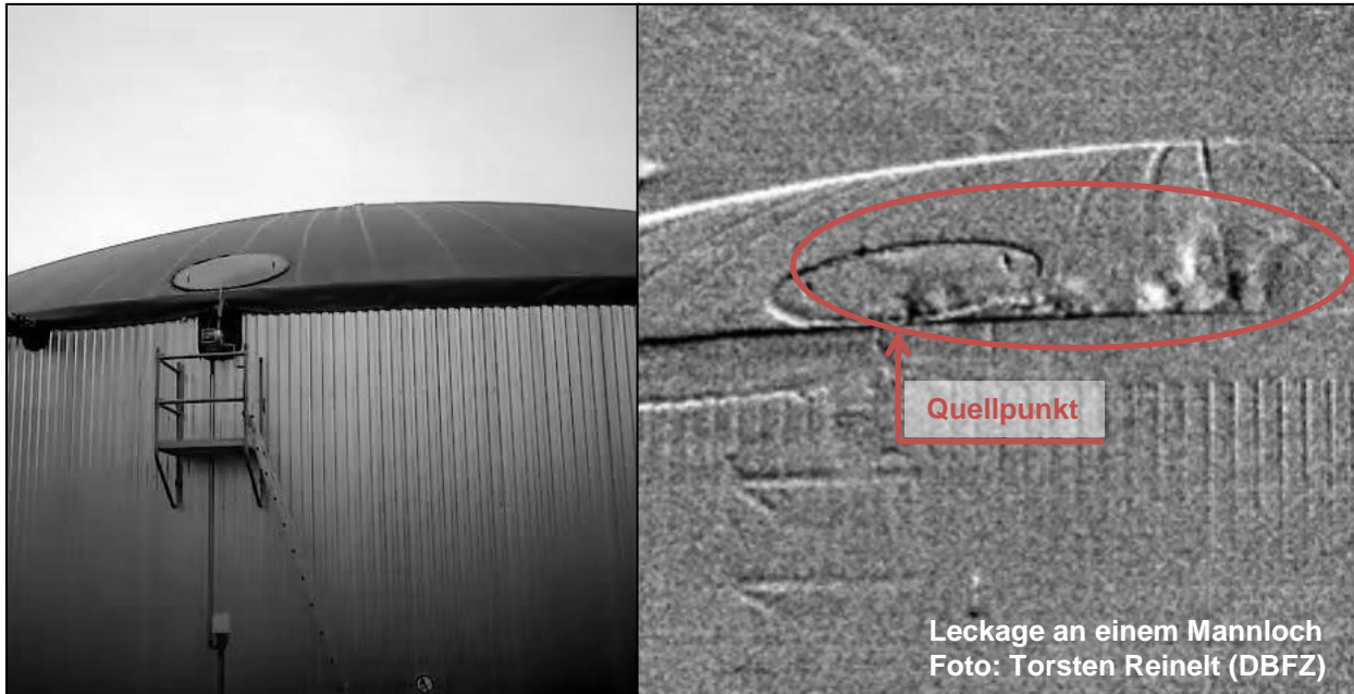
Abbildung 5-14: Leckage an einem Mannloch eines Nachgärers
