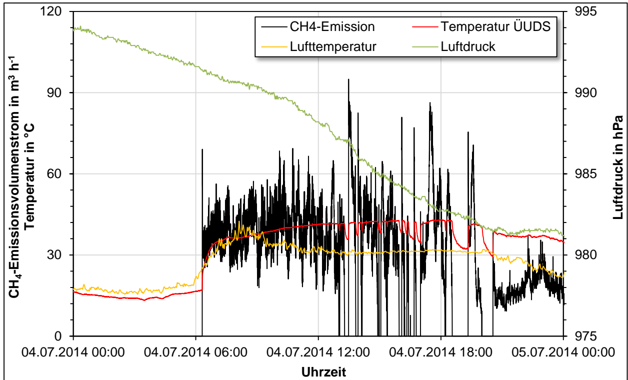
Abbildung 5-35: Tagesgang der ÜUDS am Hauptfermenter (1. Stufe) der Anlage B am 04.07.2014
