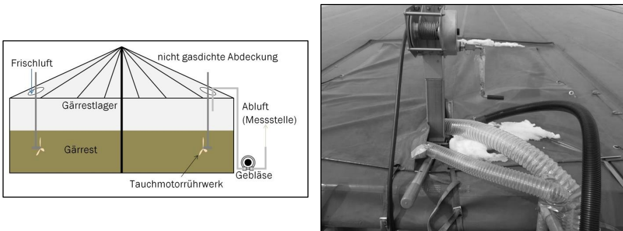
Abbildung 5-5: links im Bild: schematische Darstellung der Methodik für nicht gasdicht abgedeckte Gärrestlager; rechts im Bild: Belüftungsschläuche und beheizter Probenahmeschlauch an der Öffnung zum Tauchmotorrührwerk
