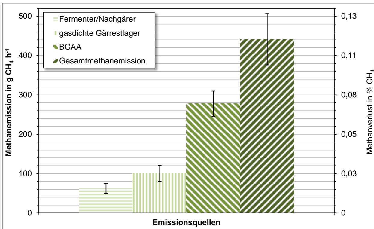
Abbildung 5-11: Methanemissionen mit Quellzuordnung in MP II der BMA I
