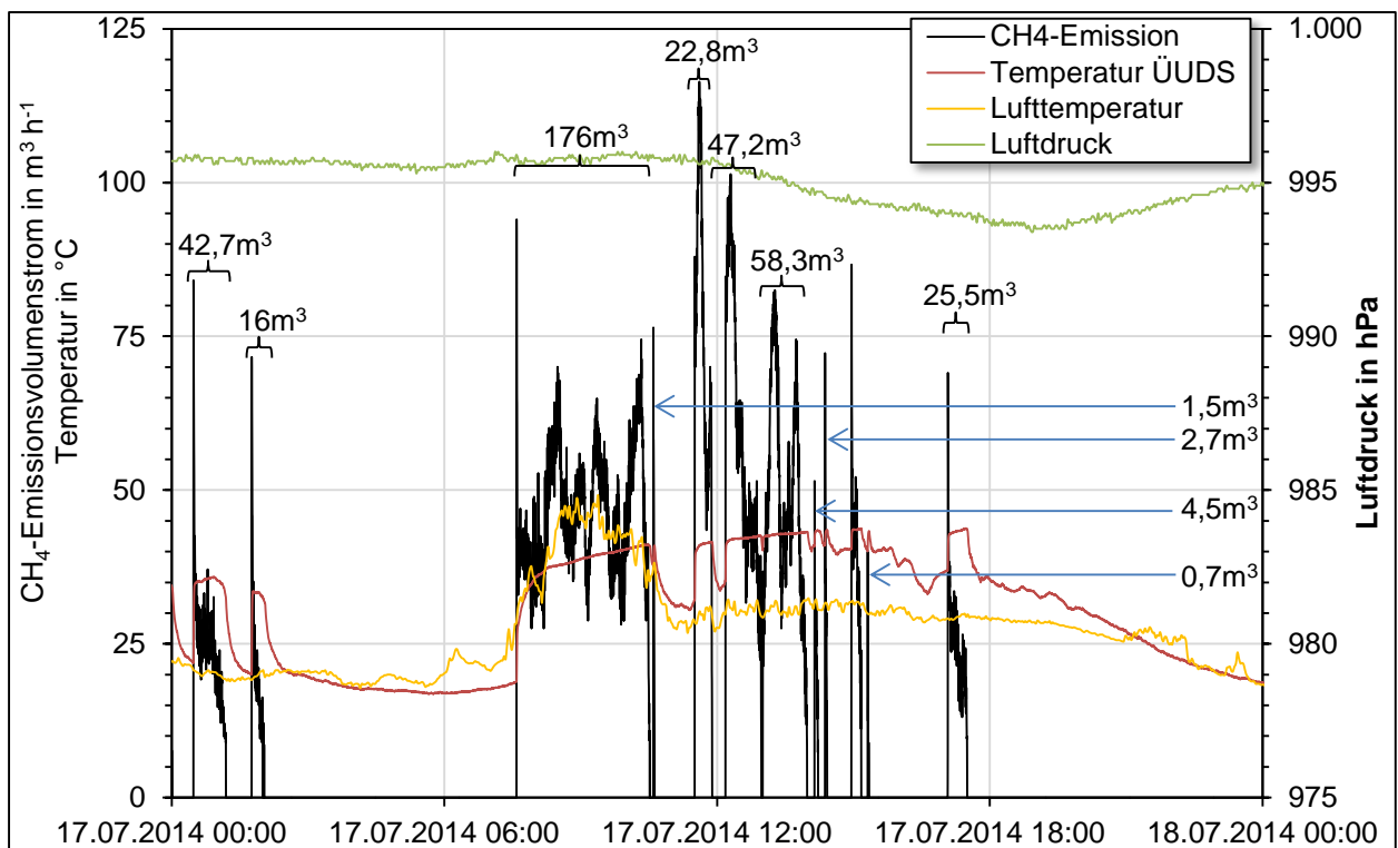
Abbildung 5-36: Tagesgang der ÜUDS am Hauptfermenter (1. Stufe) der Anlage B am 17.07.2014
