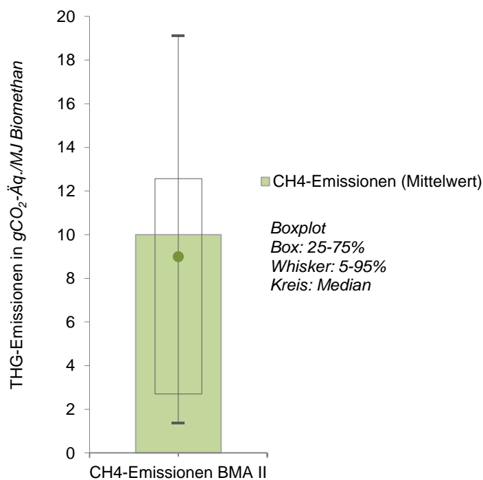
Abbildung 7-11: Treibhausgaspotential der gemessenen CH 4 -Emissionen der BMA II in gCO 2 -Äq./MJ Biomethan
