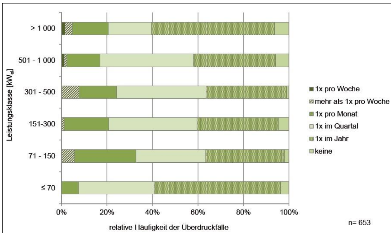
Abbildung 5-26: Häufigkeit des Auslösens von ÜUDS an Biogasanlagen in Abhängigkeit von der installierten elektrischen Anlagenleistung (Mehrfachnennungen möglich, SCHEFTELOWITZ u. a., 2014)
