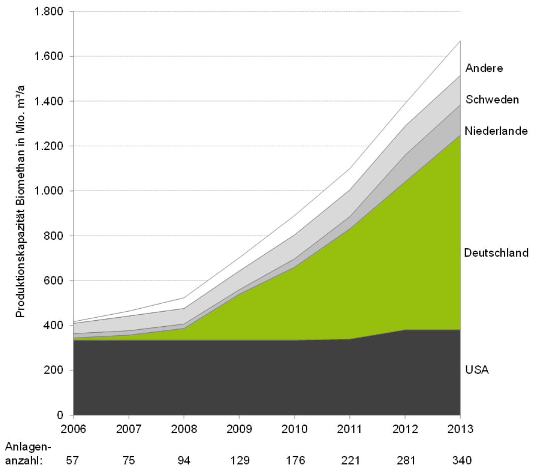
Abbildung 3-1: Entwicklung der globalen Produktionskapazität und Anlagenzahl für Biomethan bis 2013 (aus (Naumann u. a., 2014), geänderte Darstellung auf Basis von (biogaspartner, 2013; Fraunhofer IWES, 2013; IEA, 2013), © DBFZ)
