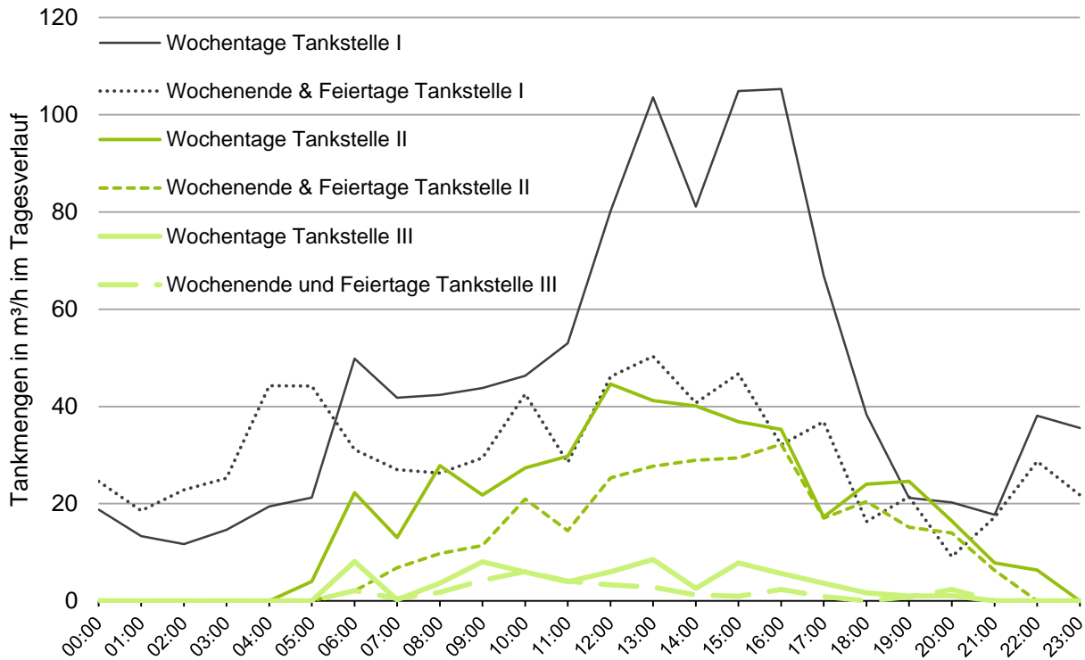
Abbildung 6-6: Stündliche Tankmengen von 3 CNG-Tankstellen (Mittelwerte Oktober 2012 bis Januar 2013)
