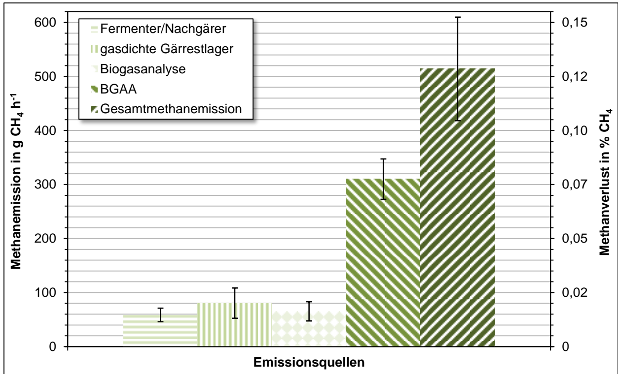
Abbildung 5-12: Methanemissionen mit Quellzuordnung in MP III der BMA I
