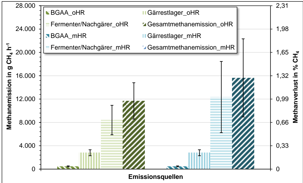
Abbildung 5-17: Mit Vor-Ort-Methode gemessene Emissionen (links) und mit Emissionsfaktoren hochgerechnete Emissionen (rechts) der MP II
