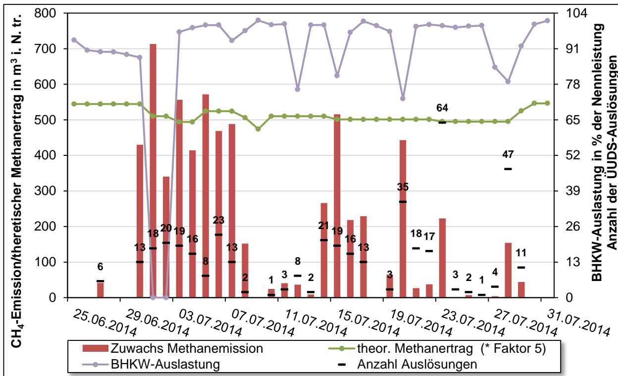
Abbildung 5-37: Überblick über den täglichen Methanverlust sowie die Anzahl registrierter Auslösungen, die BHKW-Auslastung und den theoretischen Methanertrag aus den zugeführten Substraten im Zeitraum Juni/Juli
