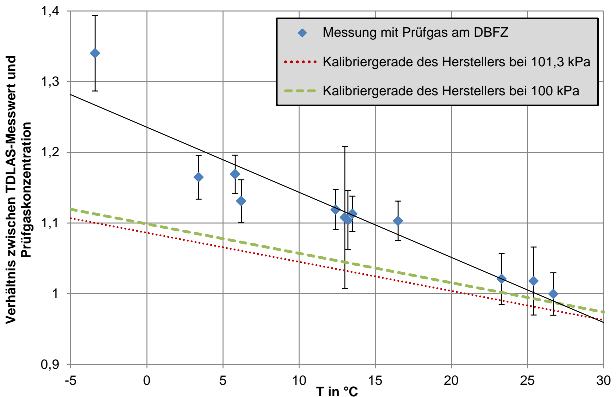
Abbildung 5-39: Temperaturkalibrierung des GasFinder CH40P-1041 (Laserspektrometer für Methan) durchgeführt mit Prüfgasen am DBFZ, Verhältnis der gemessenen Konzentration in der Gasmesszelle zur Konzentration des Prüfgases aufgetragen über der Temperatur
