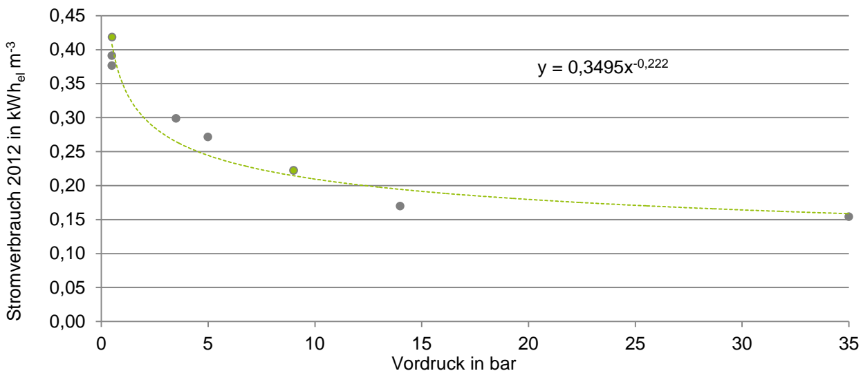
Abbildung 6-4: Spezifischer Stromverbrauch entsprechend Gasnetz-Vordruck von 8 CNG-Tankstellen der e.on (Mittelwerte 2012)
