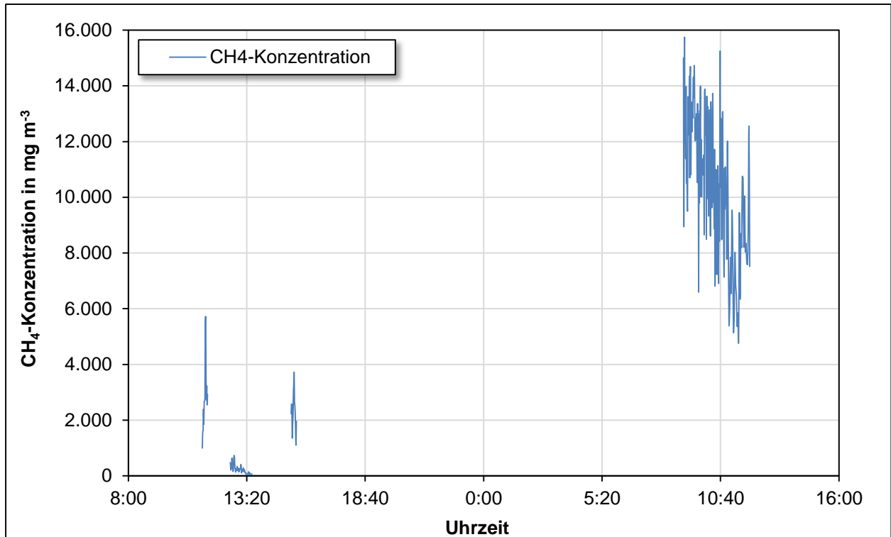
Abbildung 5-24: Langzeit-Konzentrationsverlauf der größten Leckage im Dachbereich der Hauptfermenter der BMA III
