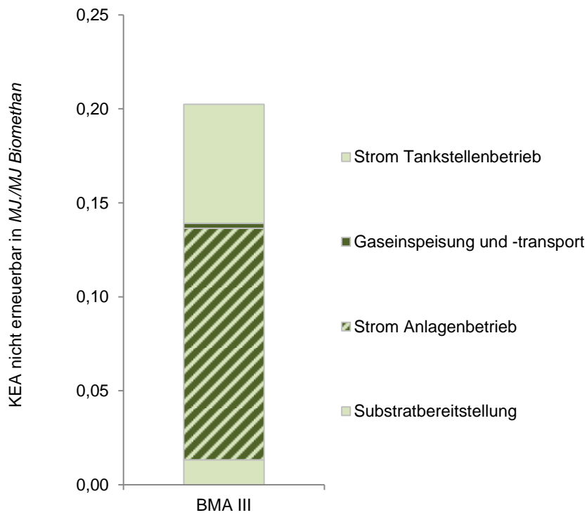
Abbildung 7-25: Kumulierter nicht erneuerbarer Energieaufwand der BMA III in MJ/MJ Biomethan
