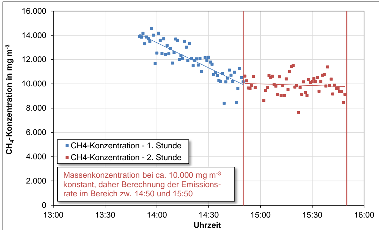
Abbildung 5-23: Konzentrationsverlauf der größten Leckage im Dachbereich der Hauptfermenter der BMA III
