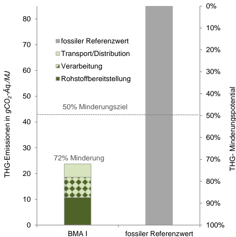
Abbildung 7-26: THG-Minderungspotenzial des in BMA I erzeugten Biomethan
