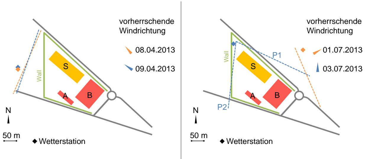
Abbildung 5-41: Schematische Darstellung des TDLAS-Messaufbaus während der Messungen im April und Juli 2013. Die gestrichelten Linien stellen die Messpfade dar. (B: Biogasanlage; A: Aufbereitungsanlage; S: Silage)
