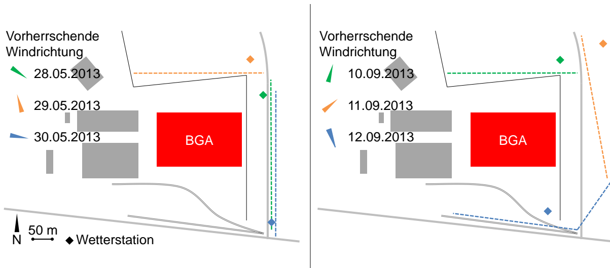
Abbildung 5-46: Schematische Darstellung des TDLAS-Messaufbaus an der BMA III während der Messungen im März, April, Mai und September 2013. Die gestrichelten Linien stellen die Messpfade dar. (BGA: Biogasanlage). Die Lage der Wetterstation ist mit der gleichen Farbe kodiert wie die Windrichtung und Messstrecke. Umliegende Gebäude sind als graue Flächen dargestellt.
