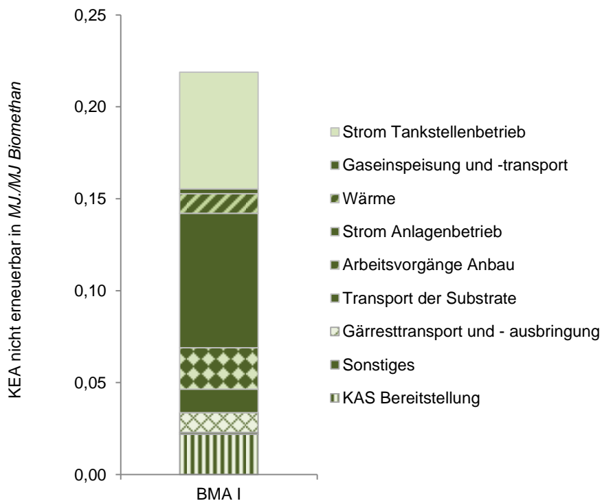
Abbildung 7-23: Kumulierter nicht erneuerbarer Energieaufwand der BMA I in MJ/MJ Biomethan
