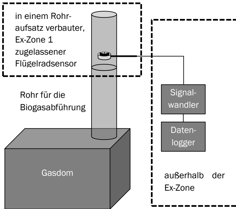
Abbildung 5-7: Schematische Darstellung der Messmethodik zur Quantifizierung austretender Methanemissionen aus ÜUDS
