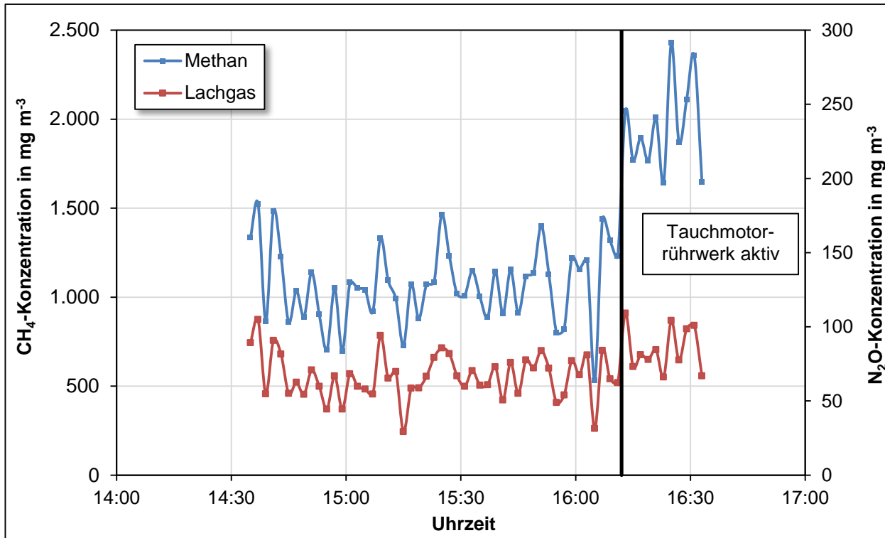
Abbildung 5-21: Einfluss von Rührintervallen auf die THG-Emission
