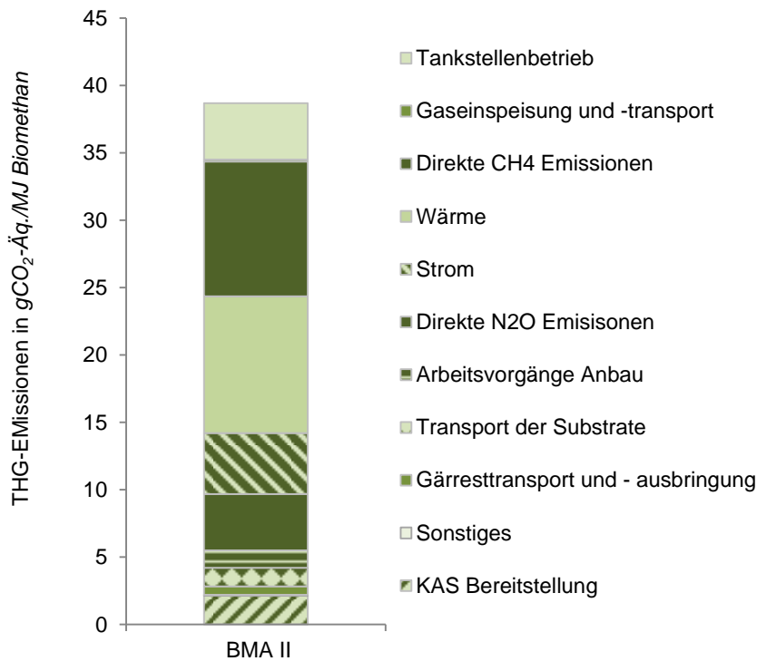
Abbildung 7-12: Gesamt THG-Emissionen der Biomethanbereitstellung der BMA II in gCO 2 -Äq./MJ Biomethan
