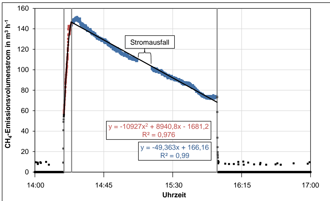
Abbildung 5-27: Auslösen der ÜUDS am Nachgärer 1 (2. Stufe) der Anlage A am 29.10.2012 infolge eines 3-stündigen Ausfalls aller verfügbaren BHKW (keine stationäre Fackel verfügbar)
