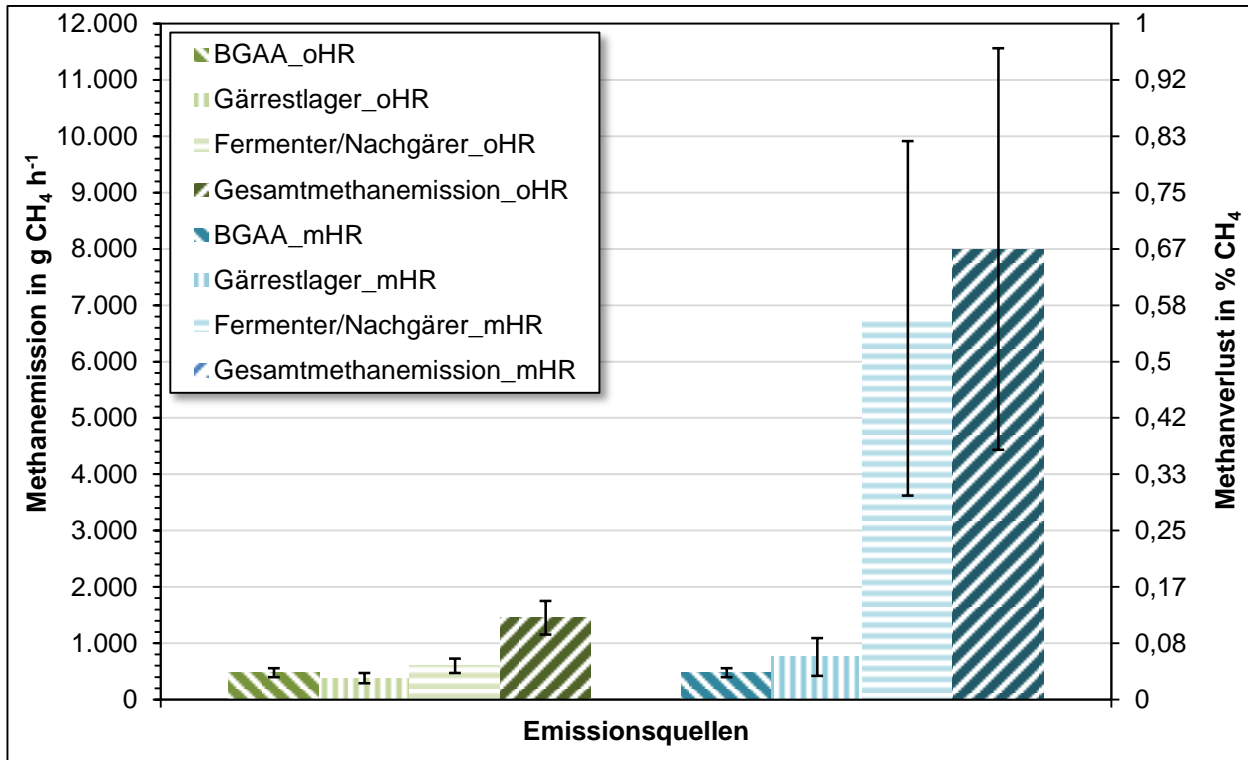
Abbildung 5-16: Mit Vor-Ort-Methode gemessene Emissionen (links) und mit Emissionsfaktoren hochgerechnete Emissionen (rechts) der MP I
