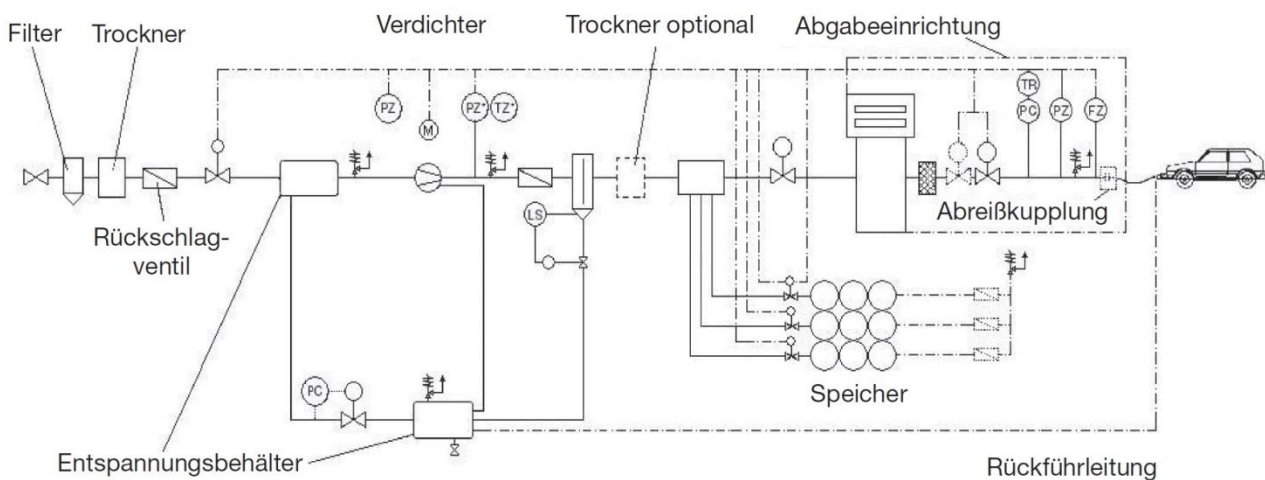
Abbildung 6-1: Schema einer Fastfill-Erdgastankstelle (Deutsche Vereinigung des Gas- und Wasserfaches e. V. (DVGW) & Verband der TÜV (VdTÜV), 2009)
