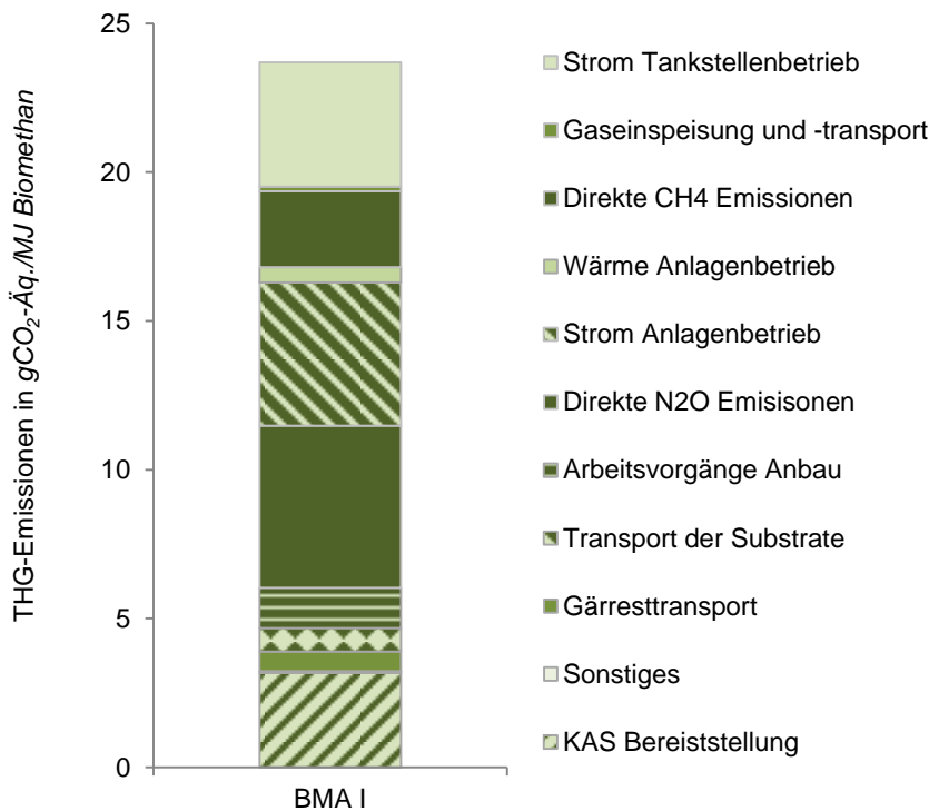
Abbildung 7-8: Gesamt THG-Emissionen der Biomethabereitung der BMA I in gCO 2 -Äq./MJ Biomethan
