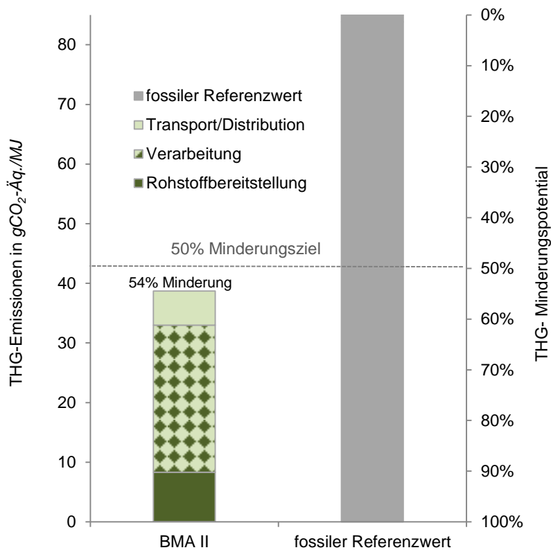
Abbildung 7-27: THG-Minderungspotential des in BMA II erzeugten Biomethan
