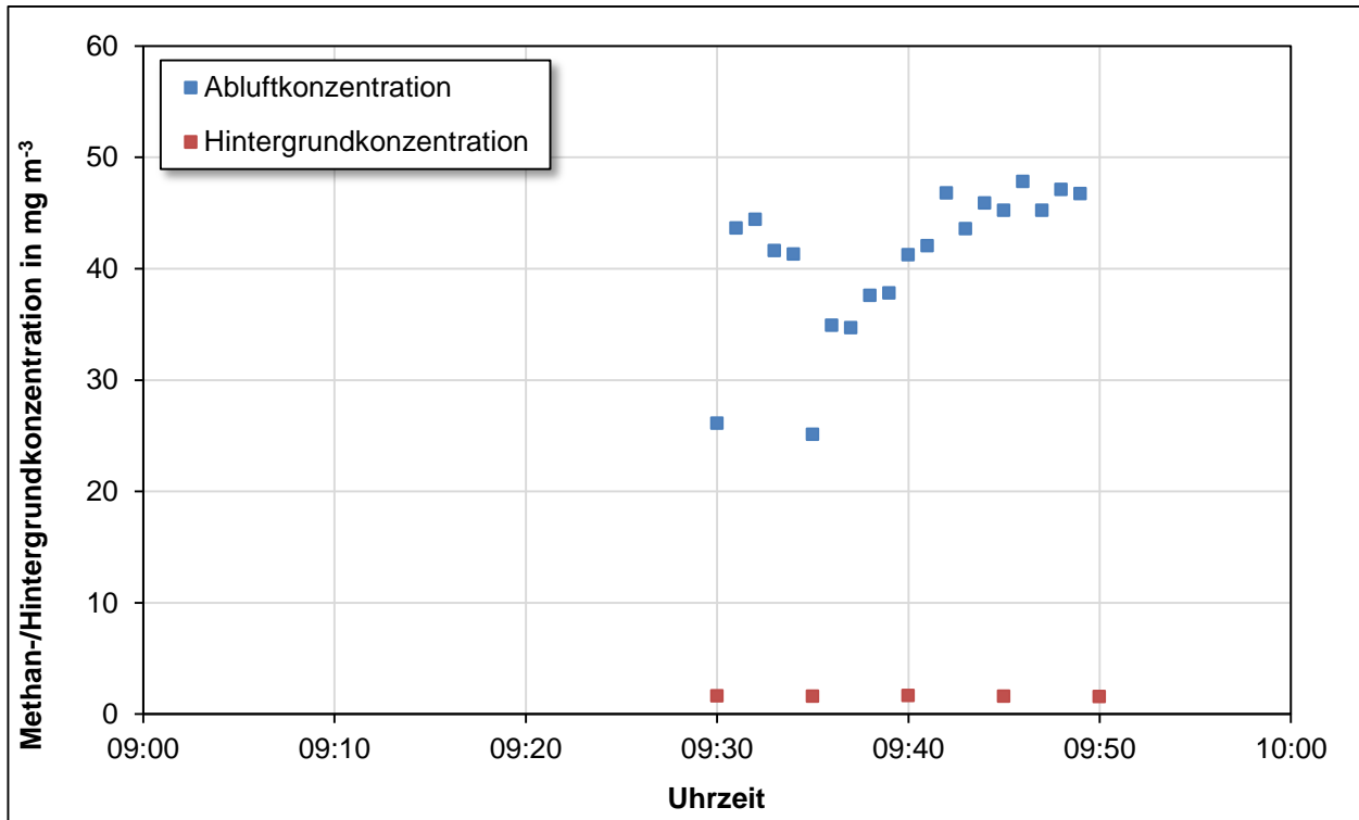
Abbildung 6-2: Verlauf der gemessenen Methankonzentration in der Abluft einer Verdichterstation einer Erdgastankstelle während einer Betriebsphase (Mai 2013; \dot{V} = 12.112 \pm 905 \text{ m}^3 \text{ h}^{-1} ; E = 476,2 \pm 119,7 \text{ g CH}_4 \text{ h}^{-1} )
