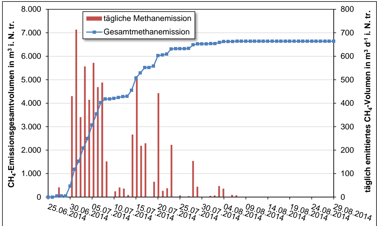
Abbildung 5-31: Entwicklung des Gesamtmethanvolumens und des täglich emittierten Methanvolumens im Messzeitraum
