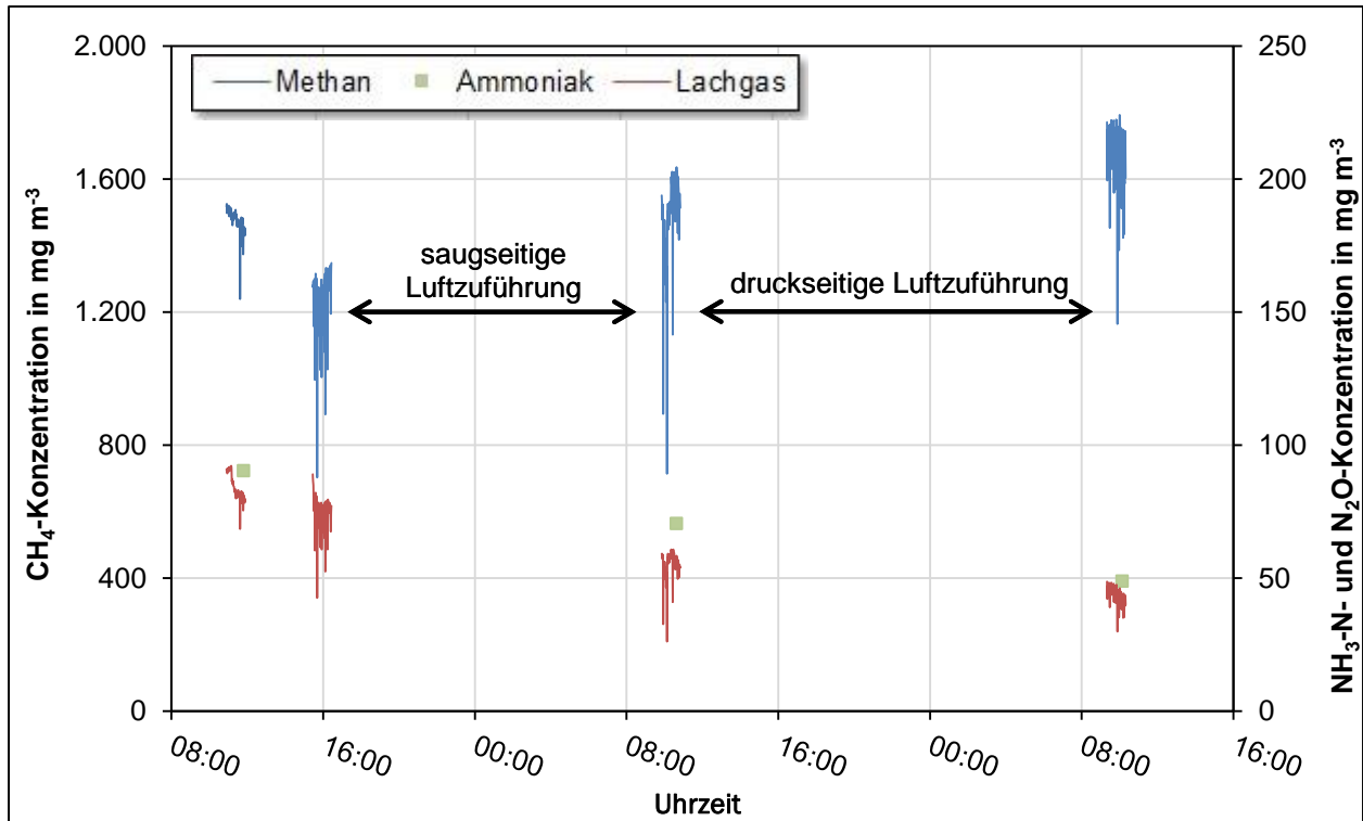
Abbildung 5-22: Langzeitmessung eines nicht gasdichten Gärrestlagers
