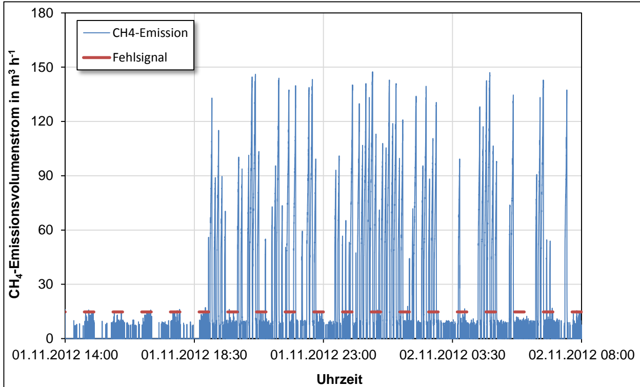
Abbildung 5-30: Auslösen der ÜUDS am Nachgärer 1 (2. Stufe) der Anlage A am 01.11. und 02.11.2012 mit unbekannter Ursache
