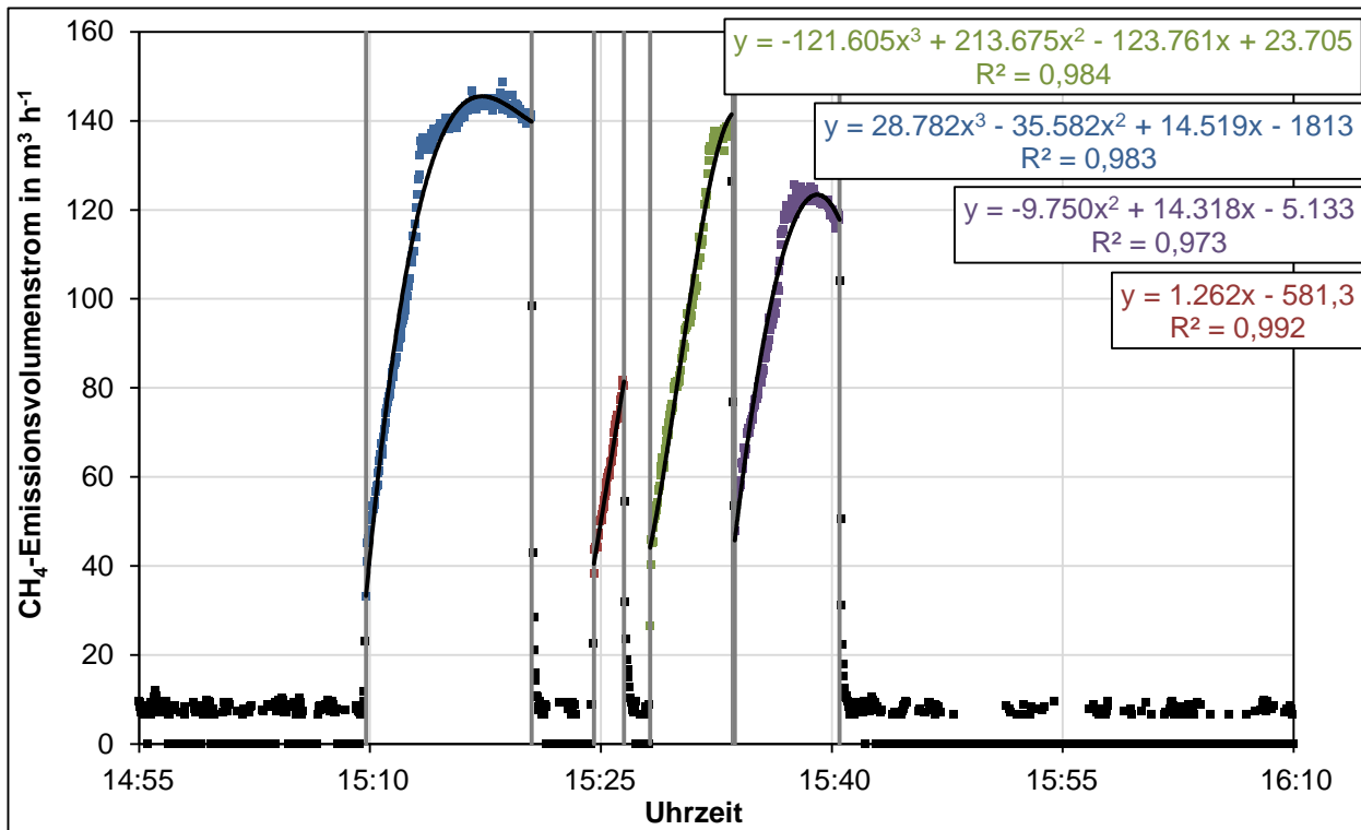
Abbildung 5-28: Auslösen der ÜUDS am Nachgärer 1 (2. Stufe) der Anlage A am 02.11.2012 infolge eines 3-stündigen Ausfalls aller verfügbaren BHKW (keine stationäre Fackel verfügbar)
