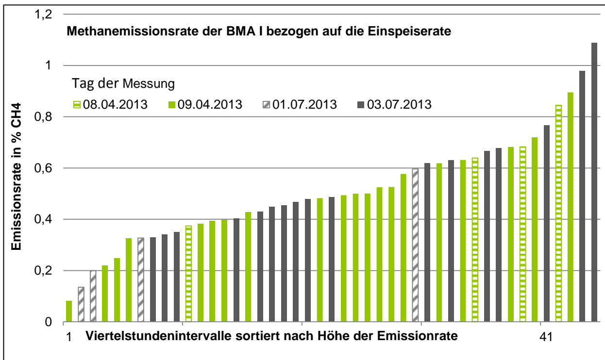
Abbildung 5-42: Emissionsraten in Viertelstunden-Werten sortiert nach der Höhe der Methan-Emission
