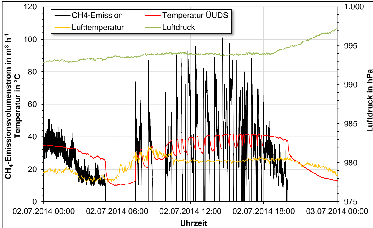
Abbildung 5-34: Tagesgang der ÜUDS am Hauptfermenter (1. Stufe) der Anlage B am 02.07.2014
