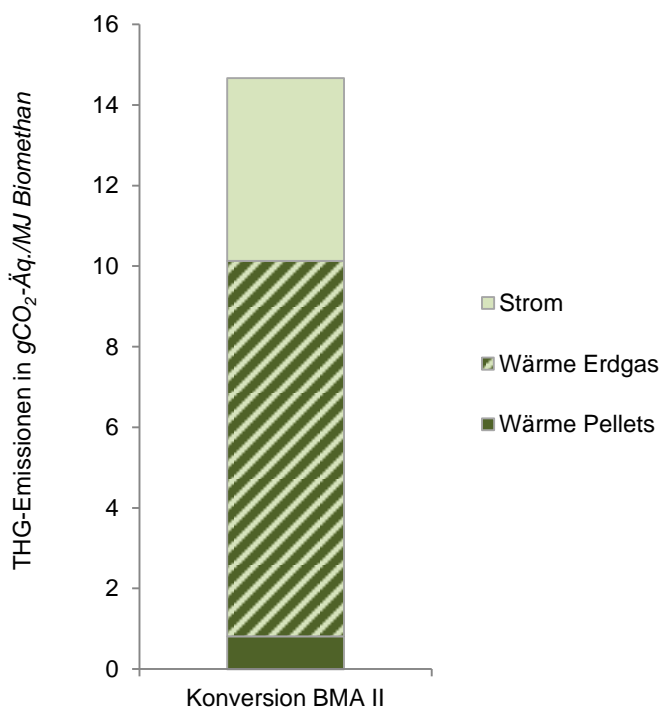
Abbildung 7-10: THG-Emissionen aus dem Anlagenbetrieb der BMA II in gCO 2 -Äq./MJ Biomethan
