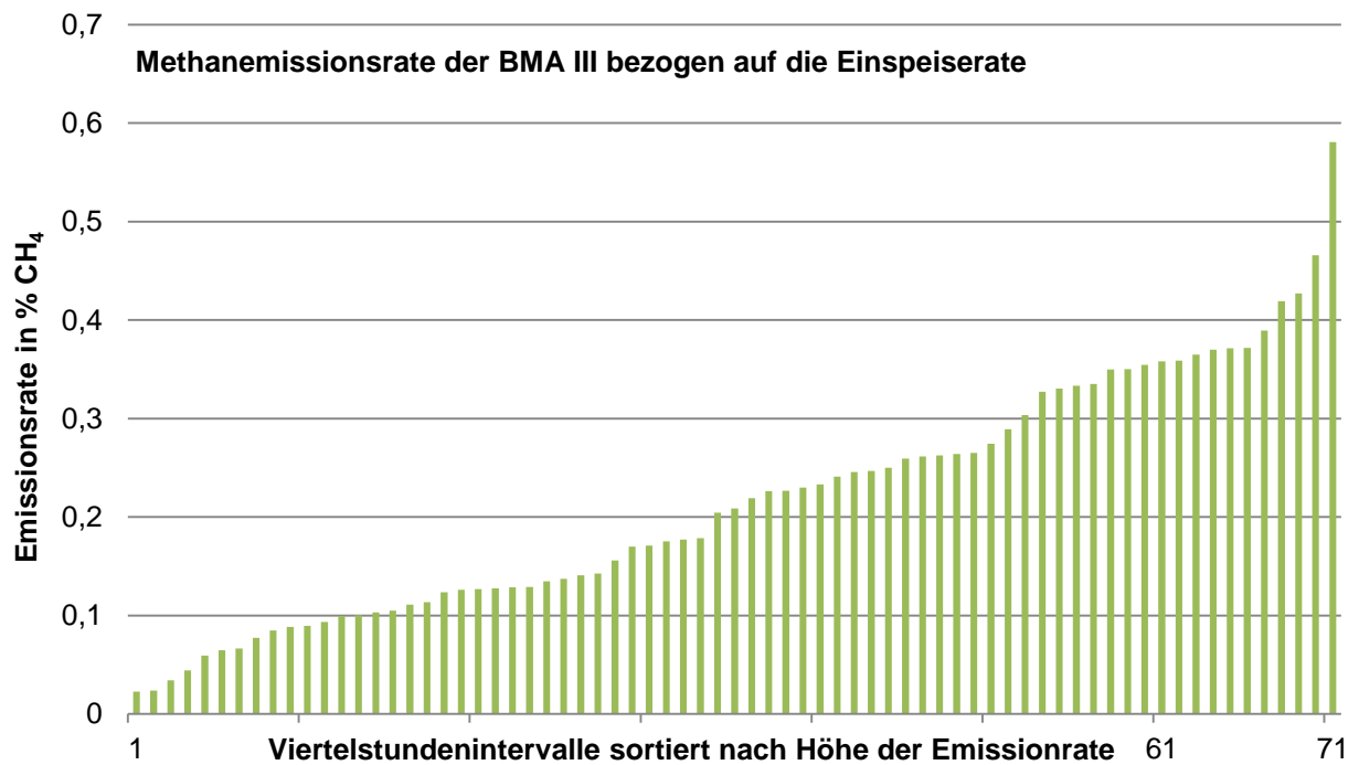
Abbildung 5-47: Emissionsraten der BMA III in Viertelstunden-Werten sortiert nach der Höhe der Methan-Emission
