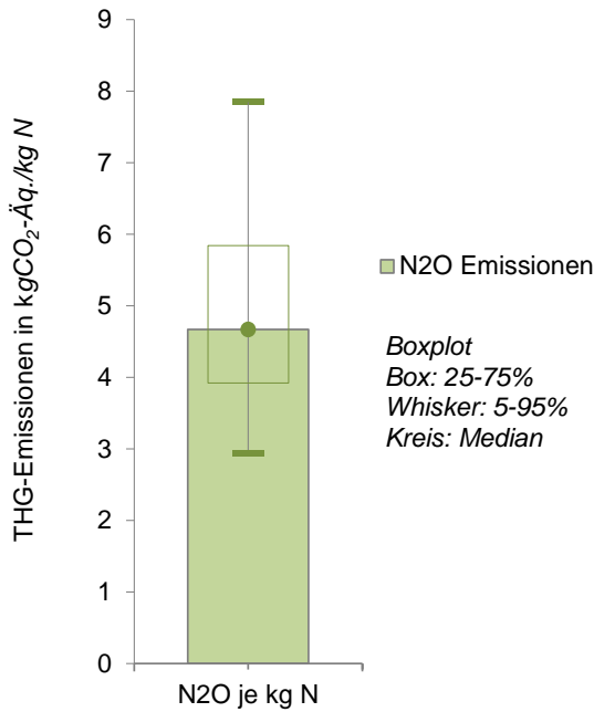
Abbildung 7-4: Ergebnisse der Monte Carlo Simulation für die direkten Lachgasemissionen
