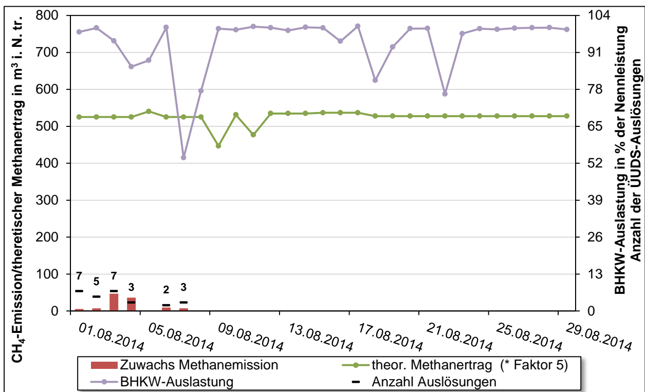
Abbildung 5-38: Überblick über den täglichen Methanverlust sowie die Anzahl registrierter Auslösungen, die BHKW-Auslastung und den theoretischen Methanertrag aus den zugeführten Substraten im Zeitraum August
